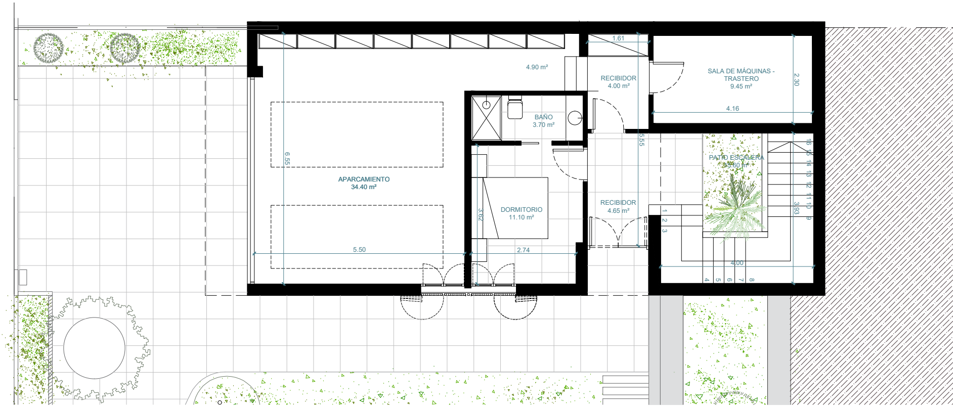
PLANTA BAJA - ACCESO
