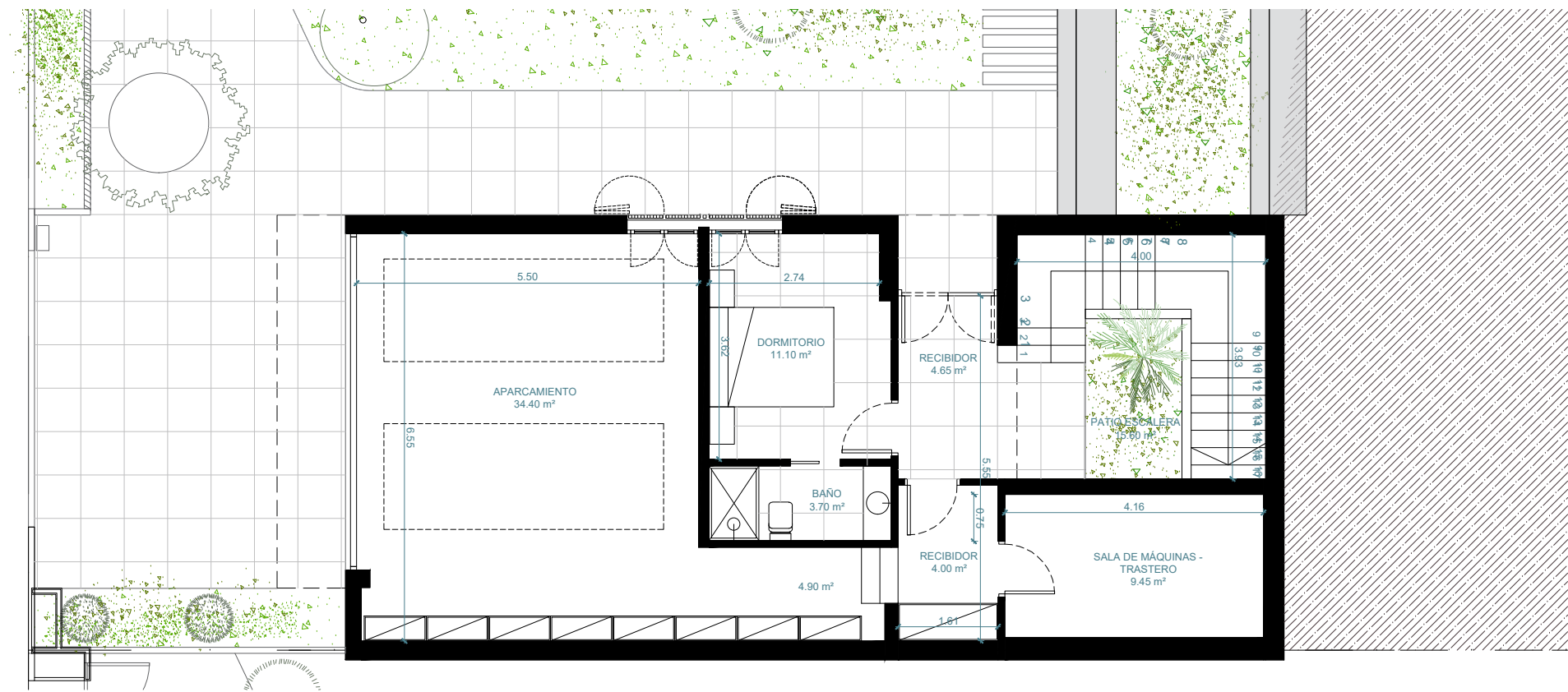
PLANTA BAJA - ACCESO
